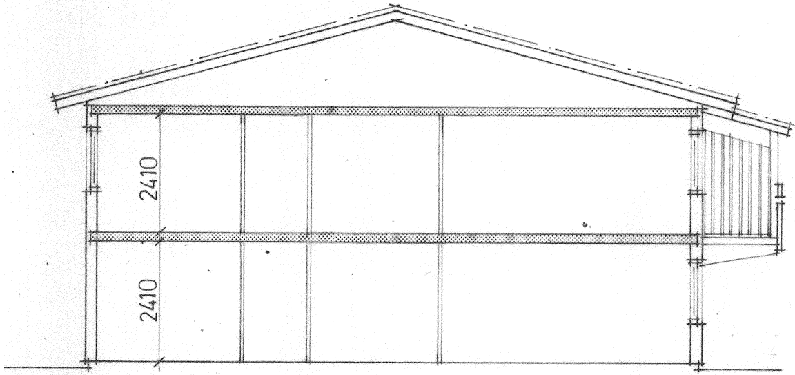
SEKTION A
