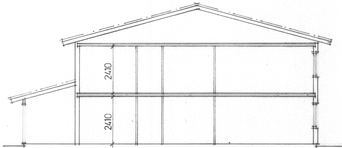
SEKTION A
