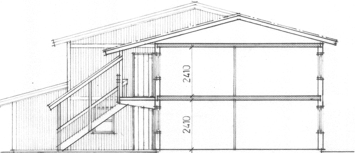
SEKTION B
