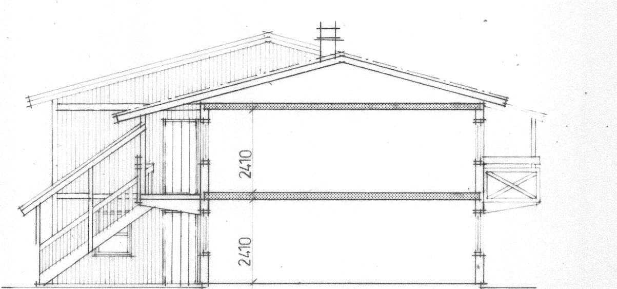
SEKTION B
