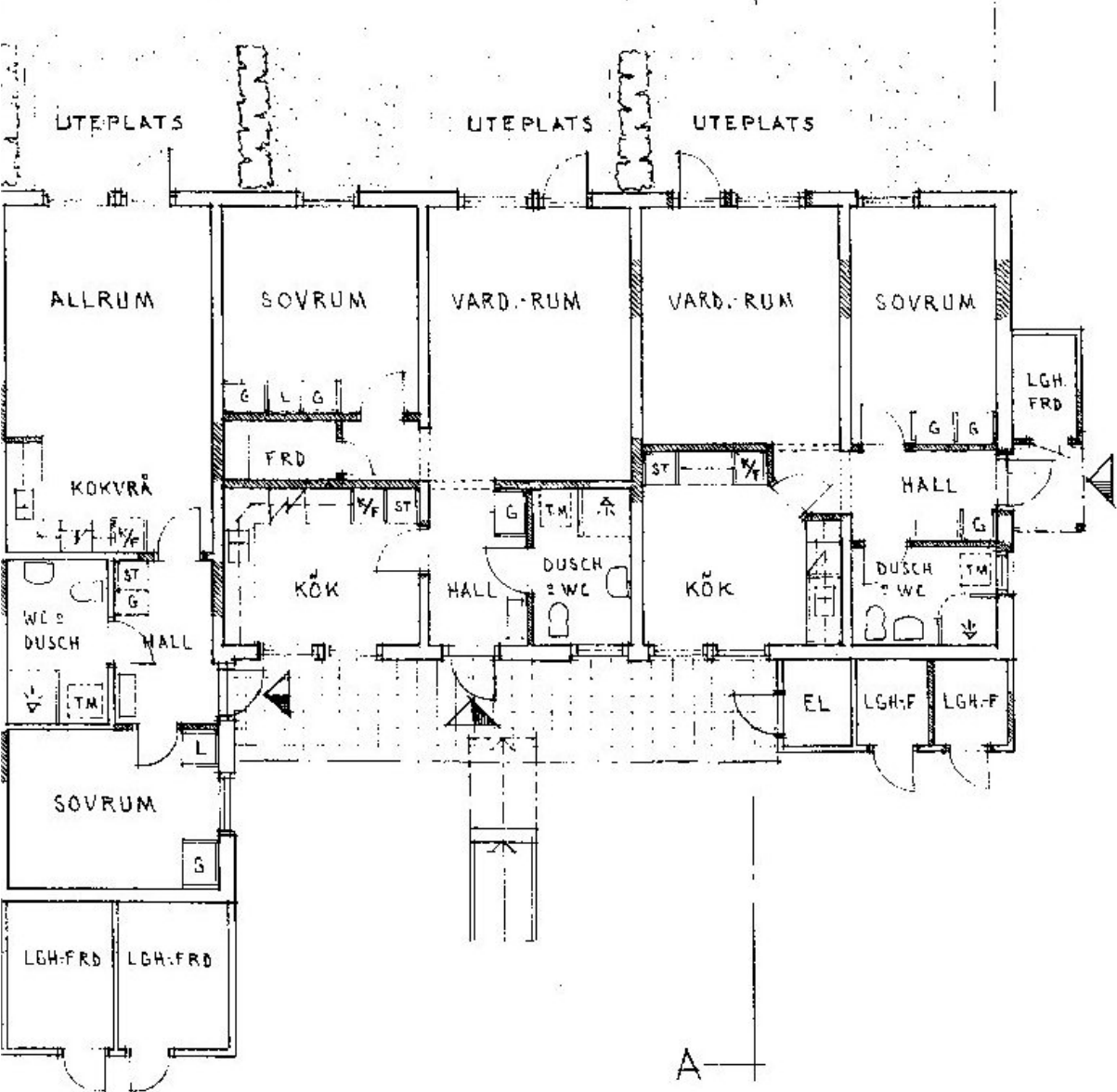
BRF VISINGE 2-rummare bottenplan där tidigare daghem
