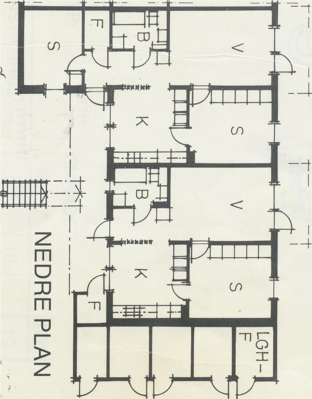
BRF VISINGE Lägenheter 3-rummare och 2-rummare bottenplan
