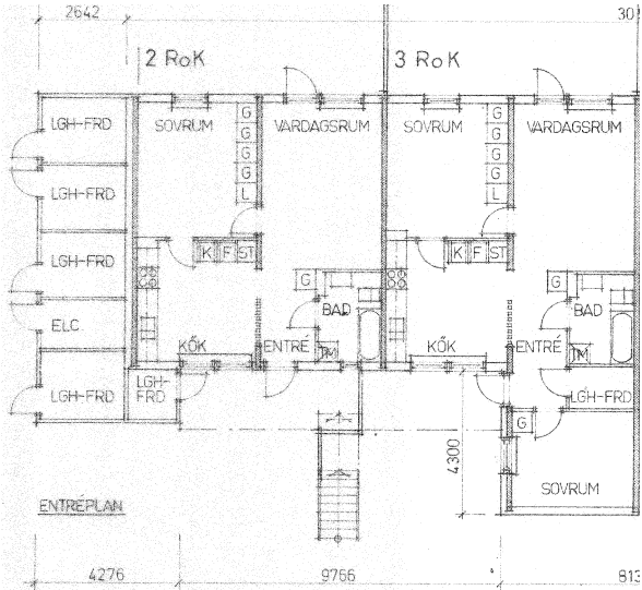
Bottenplan hus 6
